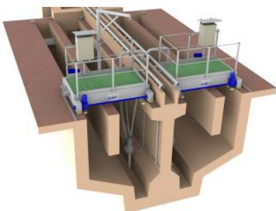
PONT DEGRAISSEUR/DESSABLEUR / GRIT AND GREASE REMOVAL BRIDGE
